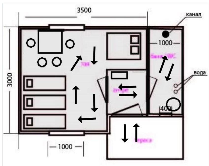
Схема за траектория на движението :
